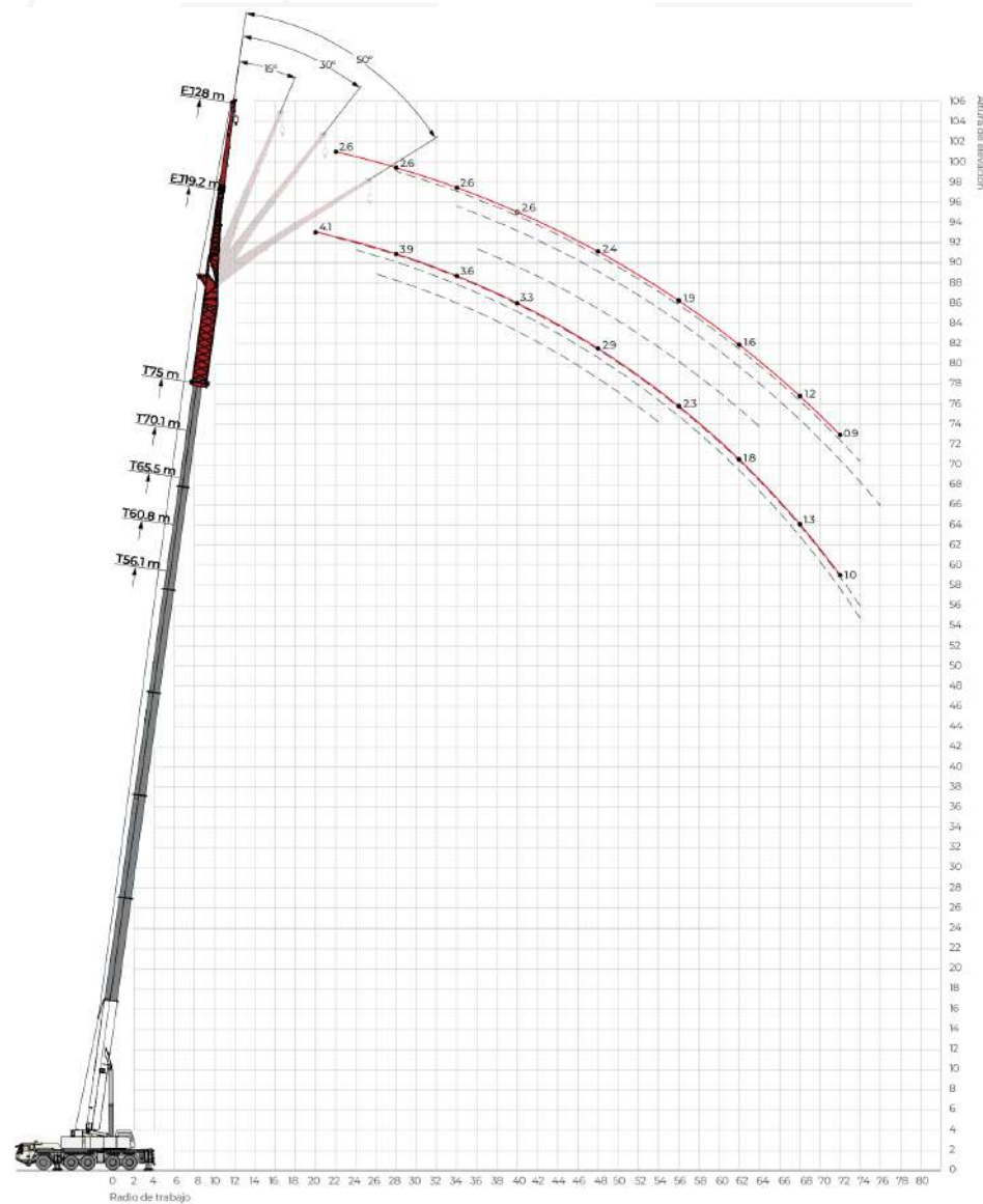
Load chart TEJ/TEH
