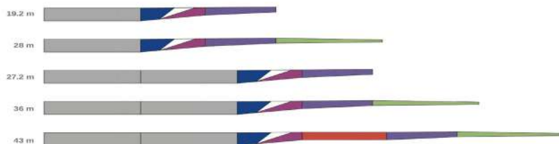
Extensión de pluma con plumín fijo Boom extension with fixed jib
