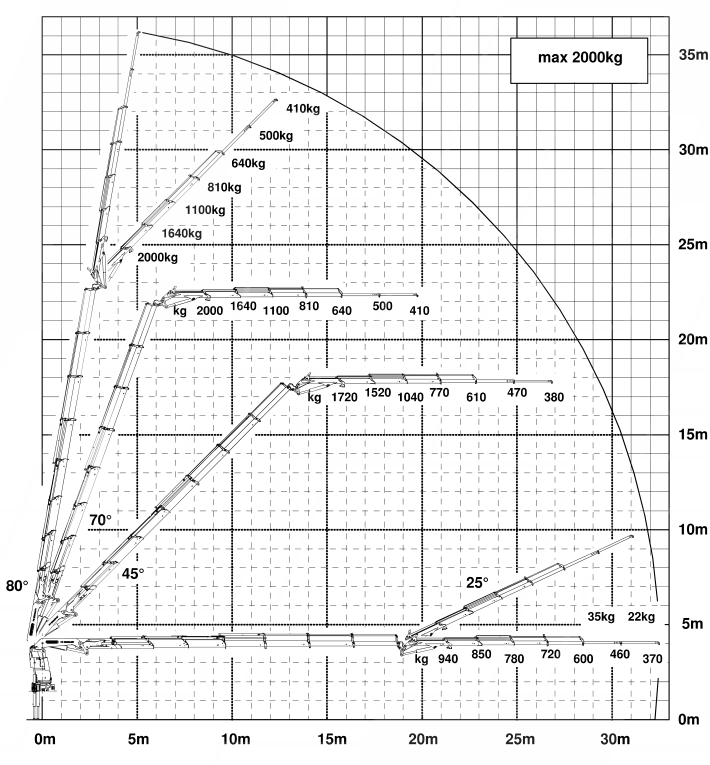
DIAGRAMA DE CARGAS CON JIB
