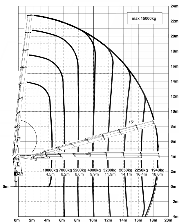
DIAGRAMA DE CARGAS
