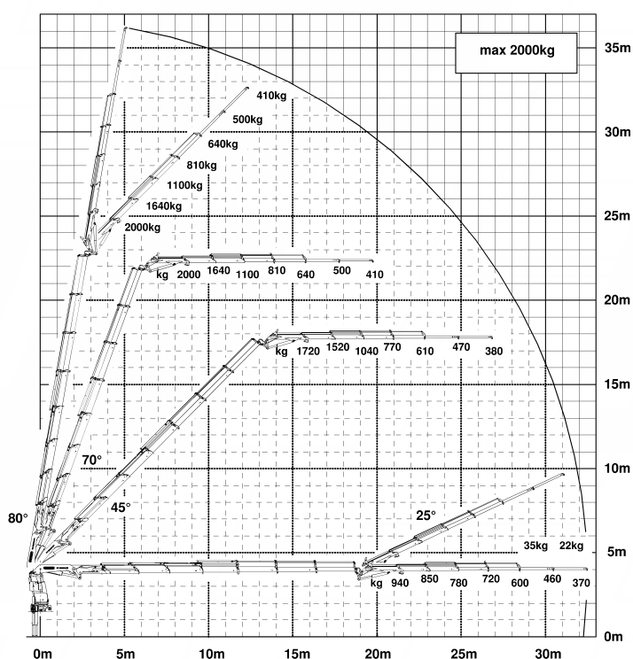
DIAGRAMA DE CARGAS CON JIB
