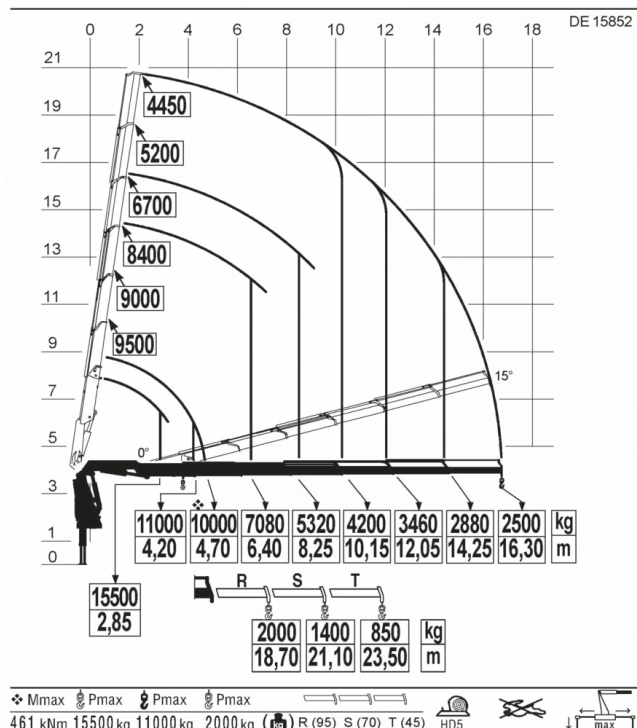
DIAGRAMA DE CARGAS
