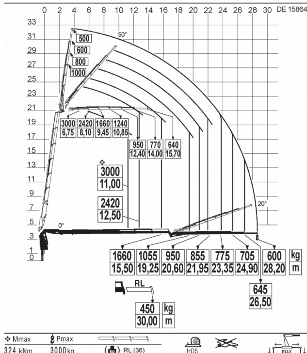
DIAGRAMA DE CARGAS CON JIB
