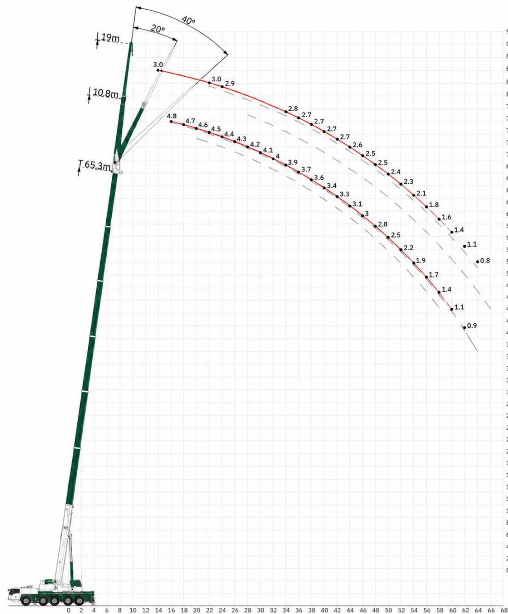
Diagrama de cargas TJ/TH
