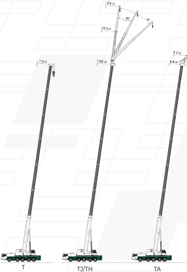
Diagrama de funcionamiento
