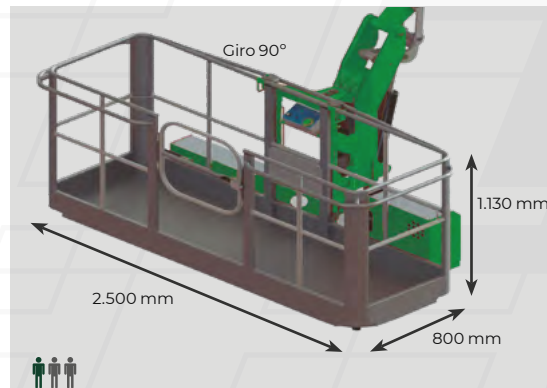
PLATAFORMA DE TRABAJO AL25E (PEMP 38 m)
