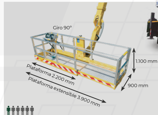
PLATAFORMA DE TRABAJO BRONTO (PEMP 56, 70, 78 Y 90 m)
